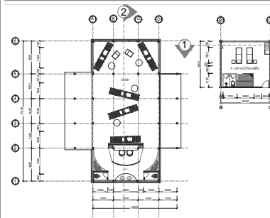
MẶT BẰNG BỐ THÍ NỘI THẤT SÁNH SPA VÀ PHÒNG TỰ LỆU DIỆN HÌNH 1/5000
