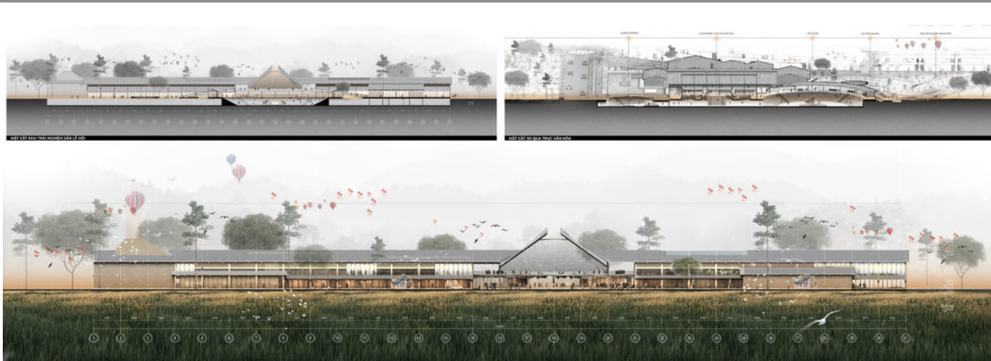
MẶT ĐỨNG - MẶT CẮT
