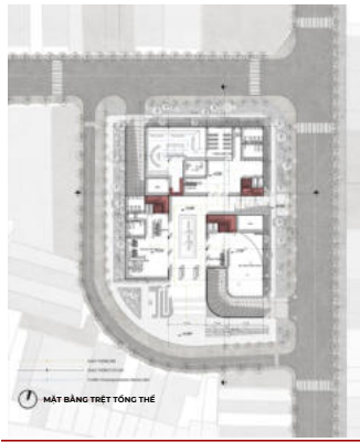
MẶT BẰNG TẦNG 1
