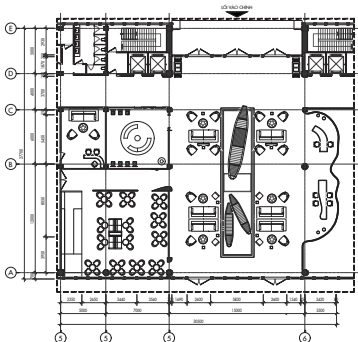
MẶT BẰNG NỘI THẤT SÂN H
