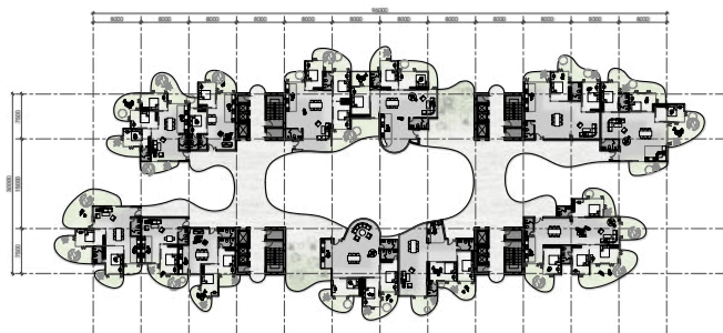
MẶT BẰNG TRIỂN KHAI CẤU TRÚC KHÔNG GIAN Ở ĐƠN NGUYÊN
