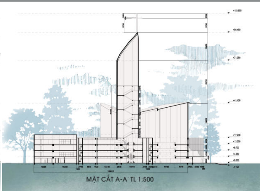
MẶT ĐỨNG - MẶT CẮT
