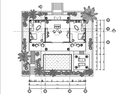
MẶT BẰNG BỐ THÍ NỘI THẤT VILLA 2 PHÒNG NGỦ 1/5000
