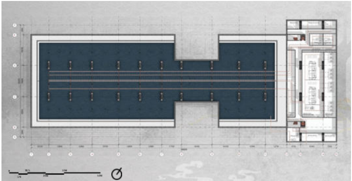
MẶT BẰNG
