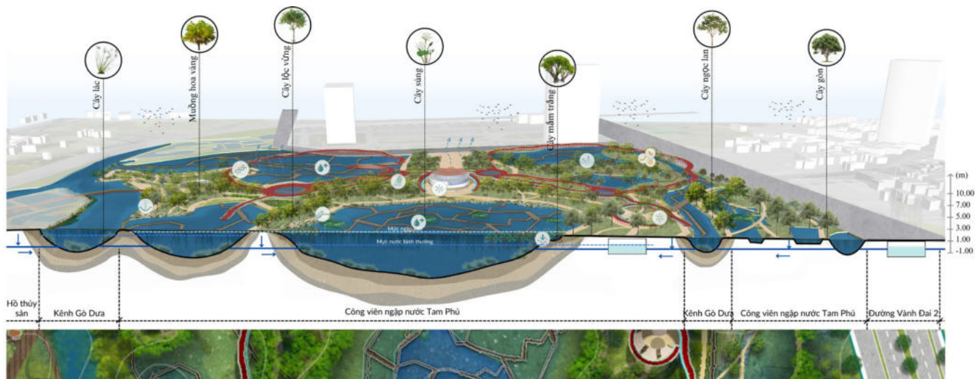
Mặt cắt ngang công viên ngập nước Tam Phú (Nguồn: Tác giả, 2024)
