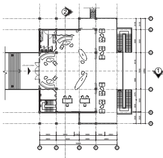
MẶT BẰNG BỐ TRÍ NỘI THẤT SÂN
