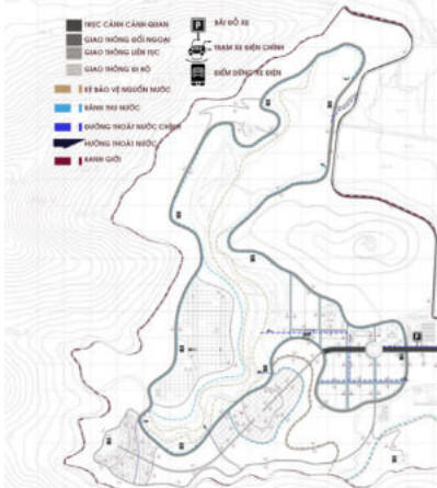
BẢN ĐỒ QUY HOẠCH GIAO THÔNG TL - 1/5000
